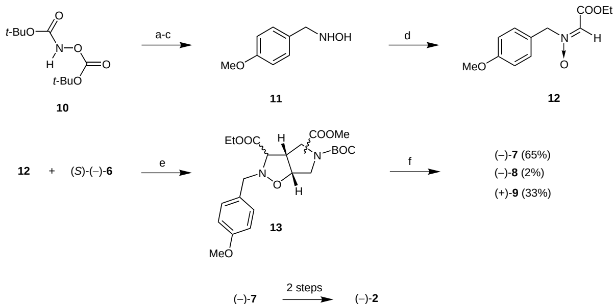
Scheme 2. (a) 4-MeOC 6 H 4 CH 2 Cl/DMF/K 2 CO 3 , 30°C; (b) TFA/CH 2 Cl 2 ; (c) aqueous K 2 CO 3 , pH 10; (d) CHOCO 2 Et, ether; (e) toluene, reflux; (f) DDQ/NEt 3 /CH 2 Cl 2 -H 2 O.
